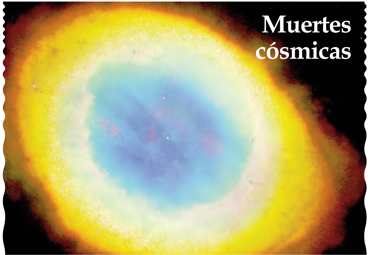
Imagen de la Nebulosa del Anillo (Ring Nebula) obtenida con el Telescopio Espacial Hubble. Crédito: Hubble Heritage Team (AURA/STScI/ NASA), tomada de http://www.phys.ncku.edu.tw/~astrolab/mirrors/apod_e/image/9901/m57ring_hst_big.jpg
